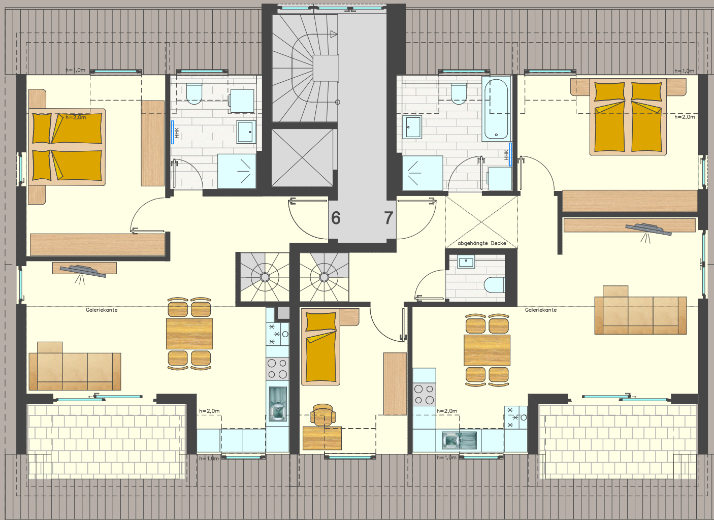
Dachgeschoss
